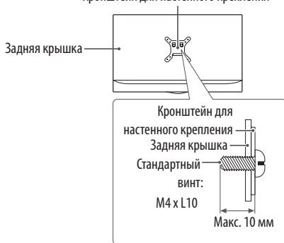
Кронштейн для настенного крепления
