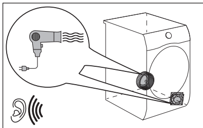
Veikia ventiliatoriai.
