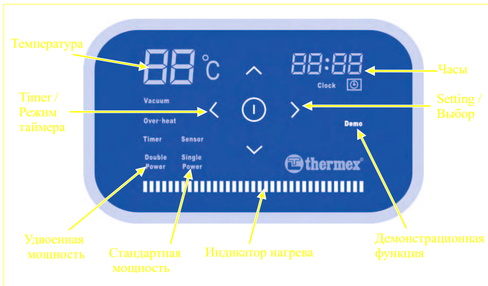
Рис. 6. Электронная панель управления (вариант 2)
