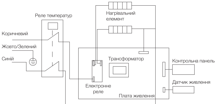
Схема електричних з'єднань для EWH Formax DL
