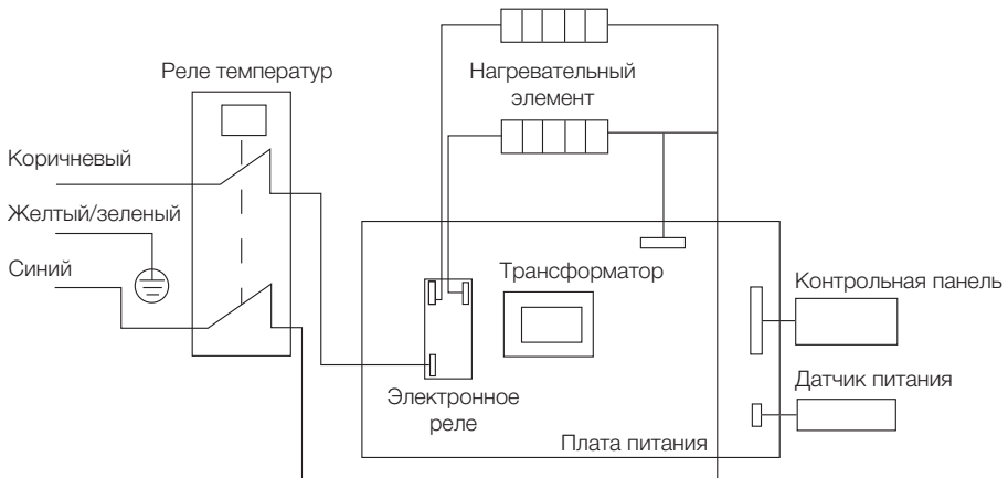
Схема электрических соединений для EWH Formax DL
