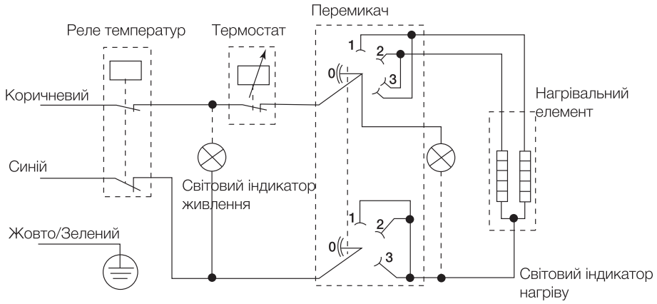
Схема електричних з'єднань для EWH Formax
