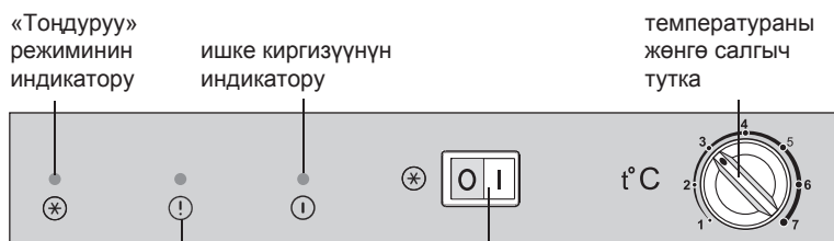
3-сүрөт – Тоңдургучтун башкаруу түзүлүштөрү
