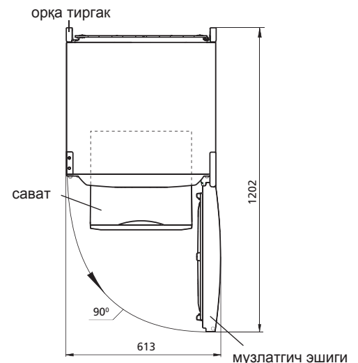
2-расм — Музлатгич (тепадан кўриниш)
