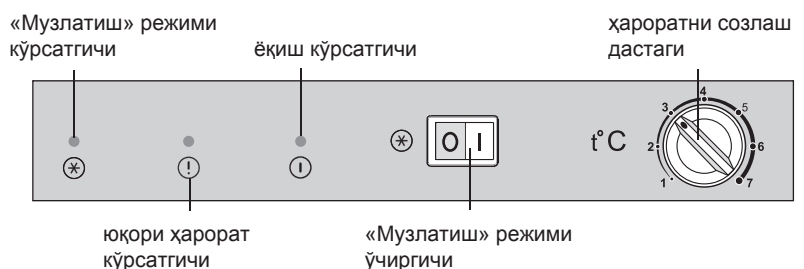
3-расм — Музлатгични бошқариш мосламалари
