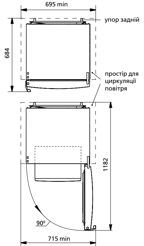
Рисунок 2 – Морозильник (вигляд зверху)
